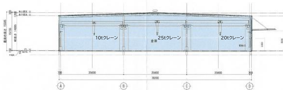
断面図_A
