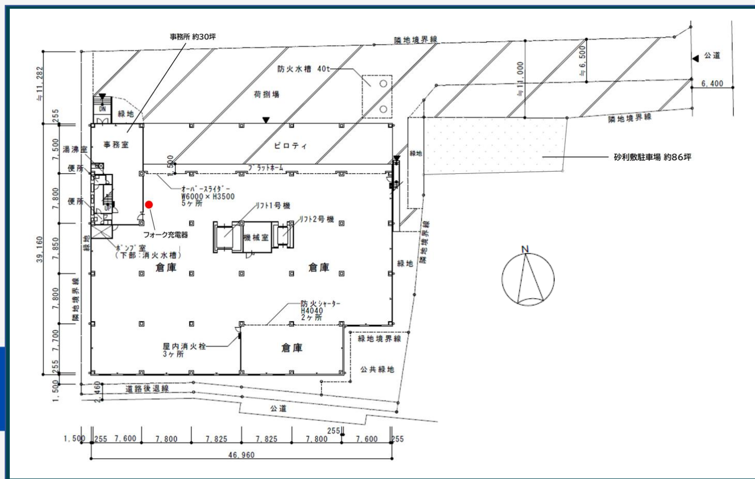
配置図・1階平面図
